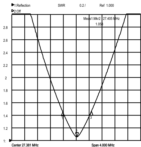
VSWR
