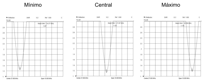
VSWR
